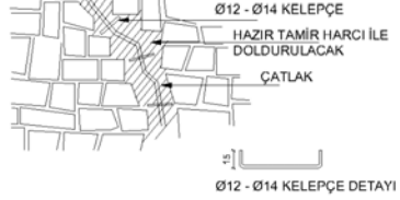
TAŞ DUVARDA ÇATLAK ONARIMI
