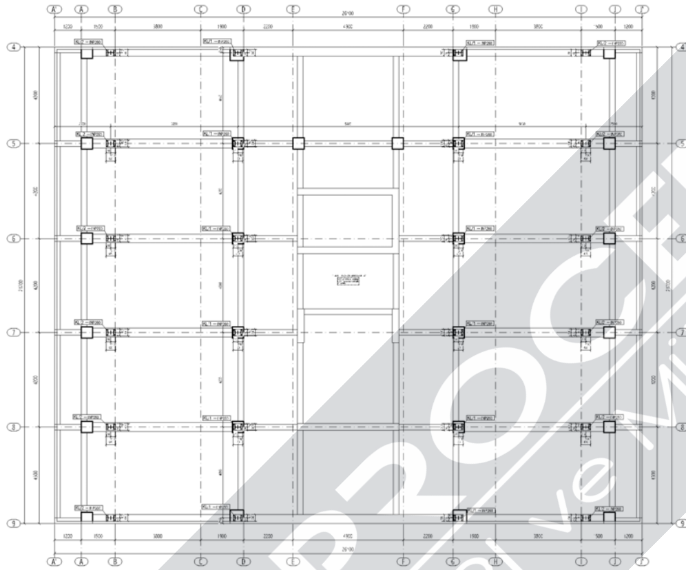
CATI KATI İNÖN APLİKASYON PLANI (1/50)-(11/25)
