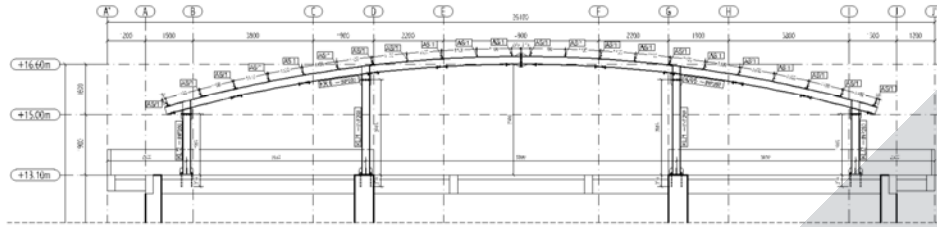
"4-4" AKSI KEŞİT GÖRÜNÜŞÜ (1/50)
