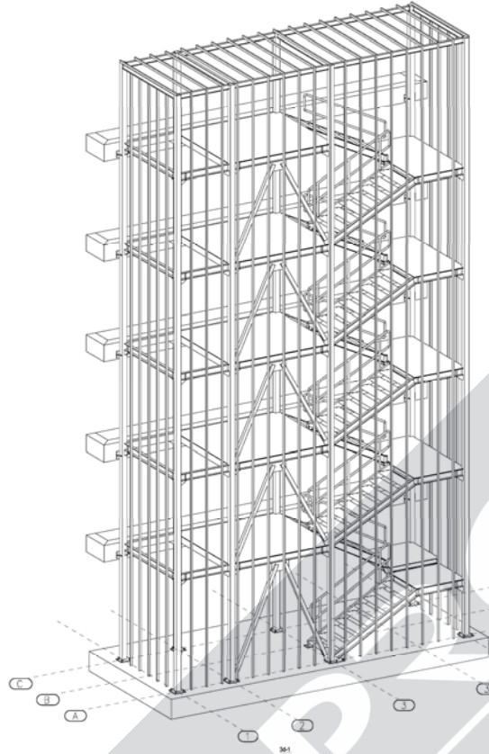
IZOMETRIK GORUNUS-1 ÖLÇEK:1/50
