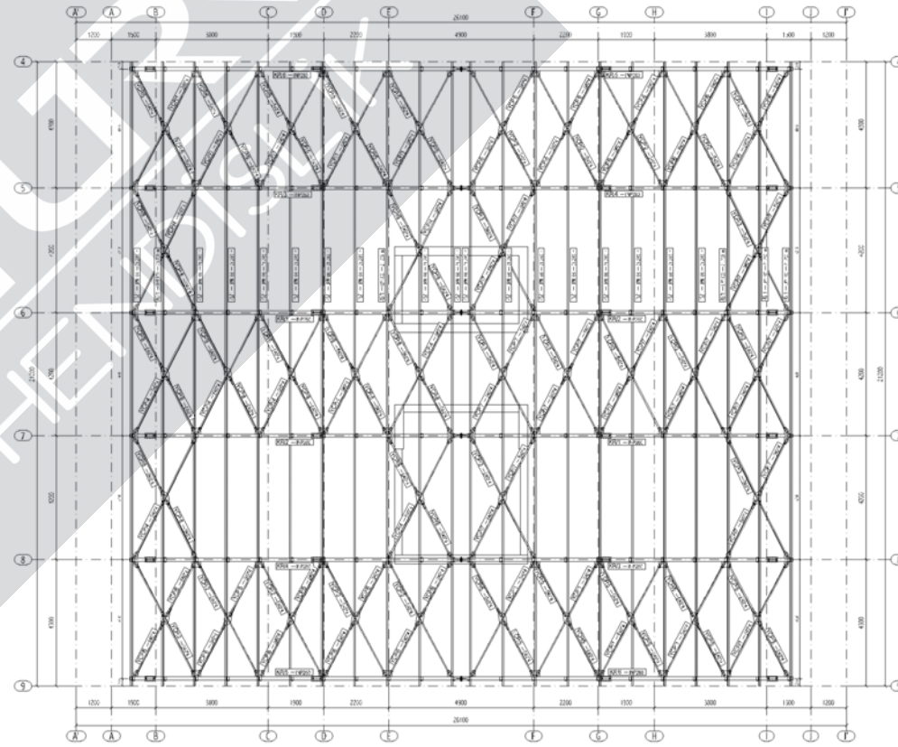
5.ETEN GÖRÜNÜŞİ (1/50)
