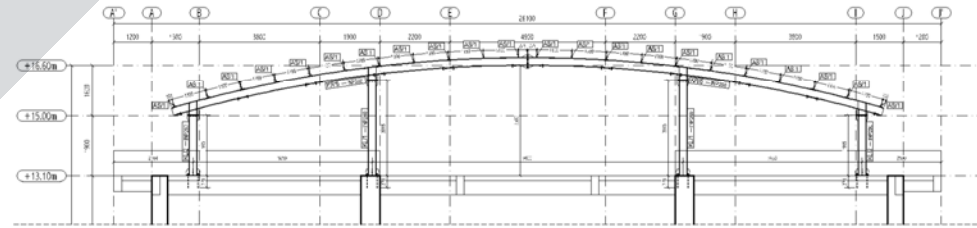
"9-9" AKSI KEŞİT GÖRÜNÜŞÜ (1/50)
