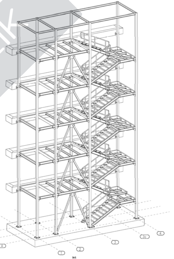
IZOMETRIK GORUNUS-3 ÖLÇEK:1/50
