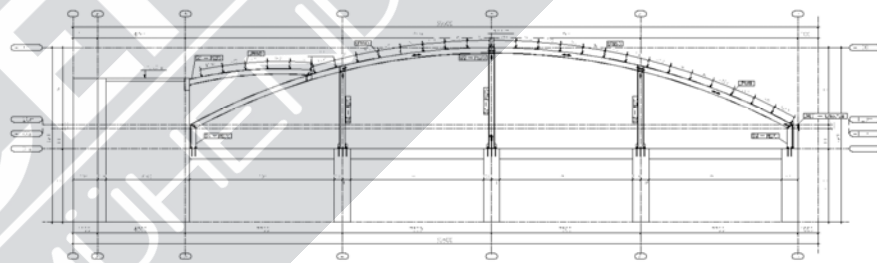
G-G AKS GÖRÜNÜŞÜ ÖLÇEK 1/50
