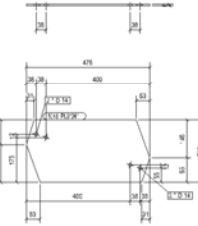
b1-b1 KESİTİ 0:1/10
