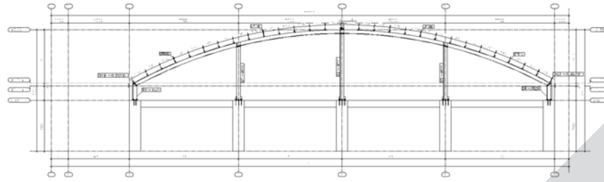
A-A AKS GÖRÜNÜŞÜ ÖLÇEK 1/50
