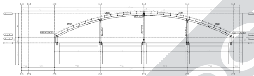
B-B AKS GÖRÜNÜŞÜ ÖLÇEK 1/50
