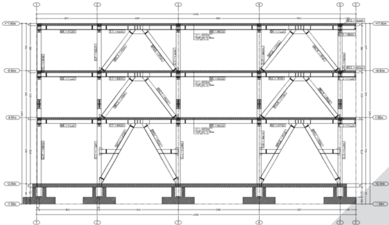
"A-A" ANI KEŞİT GÖRÜNÜŞÜ (1/50)
