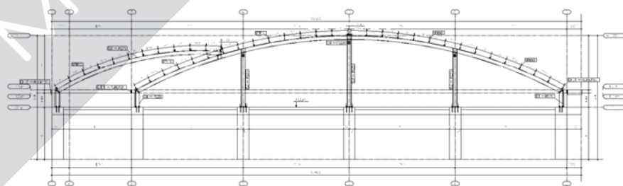
H-H AKS GÖRÜNÜŞÜ ÖLÇEK 1/50
